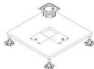
Dimensioni (AxB) 145 x 145 mm
